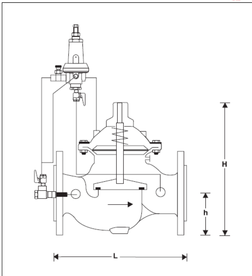
Rys. 2. Wymiary zaworu bezpieczeństwa SV300/G
