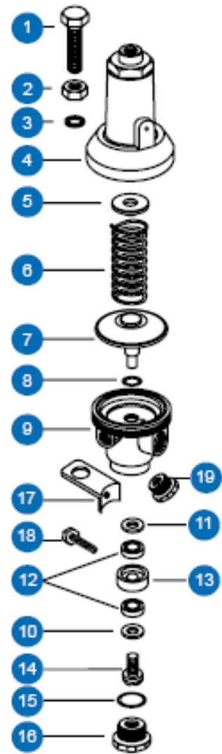
Rys. 6. Rysunek zestawieniowy zaworu sterującego 66-300
