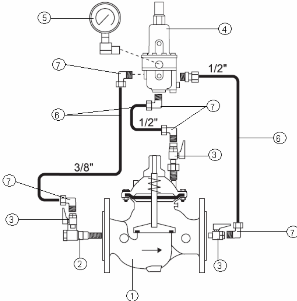
Rys. 7. Schemat połączeń zaworu bezpieczeństwa SV300/G
