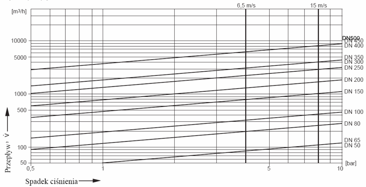
Rys. 3. Charakterystyka zaworu bezpieczeństwa SV300/G
