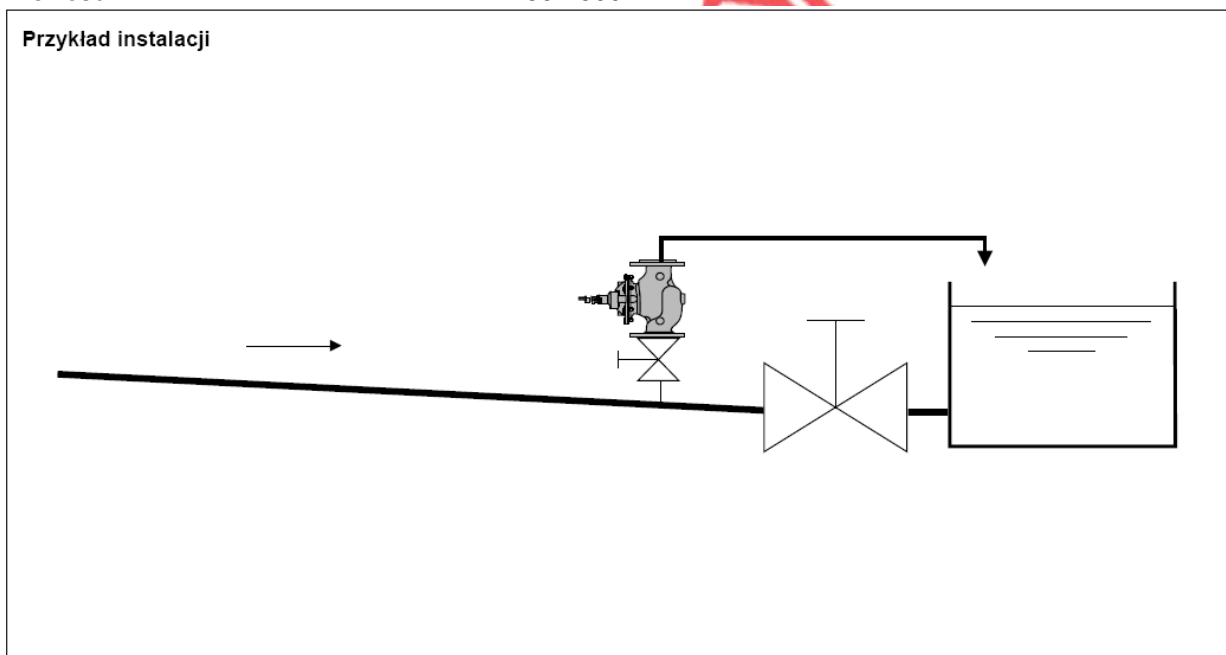
Rys. 1. Przykład instalacji z zaworem bezpieczeństwa SV300/G
