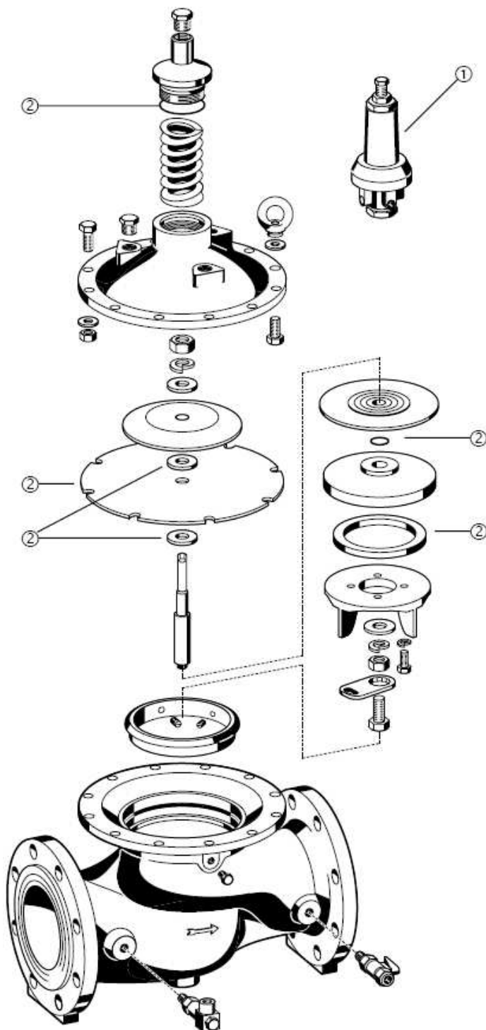
Rys. 8. Wykaz części zamiennych zaworu bezpieczeństwa SV300/G
