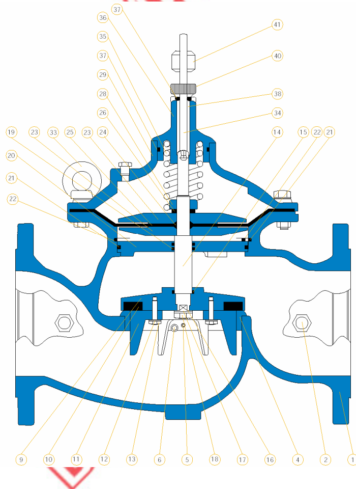
Rys. 4. Rysunek przekrojowy zaworu bezpieczeństwa SV300/G
